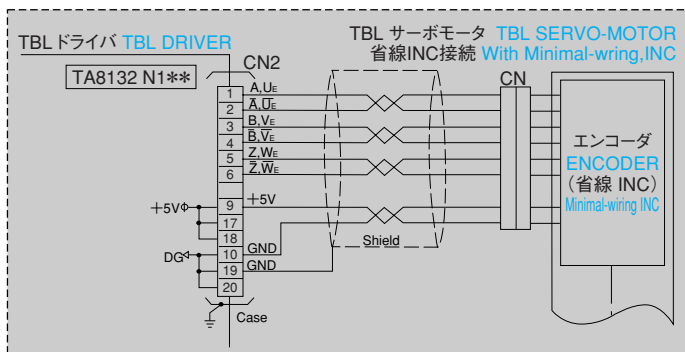
センサタイプ別接続 Sensor type-specific connections
