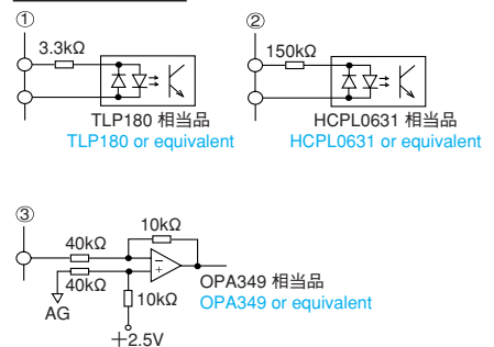
出力回路 Output circuit
