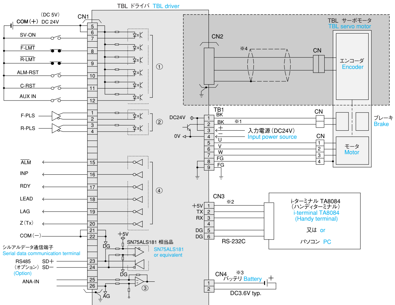
エンコーダタイプ別接続 Encoder type-specific connections
