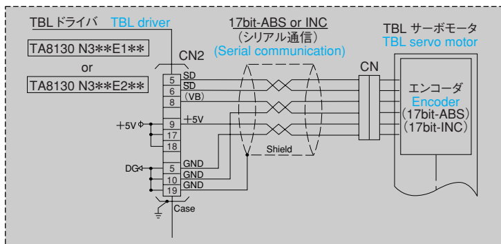
エンコーダタイプ別接続 Encoder type-specific connections
