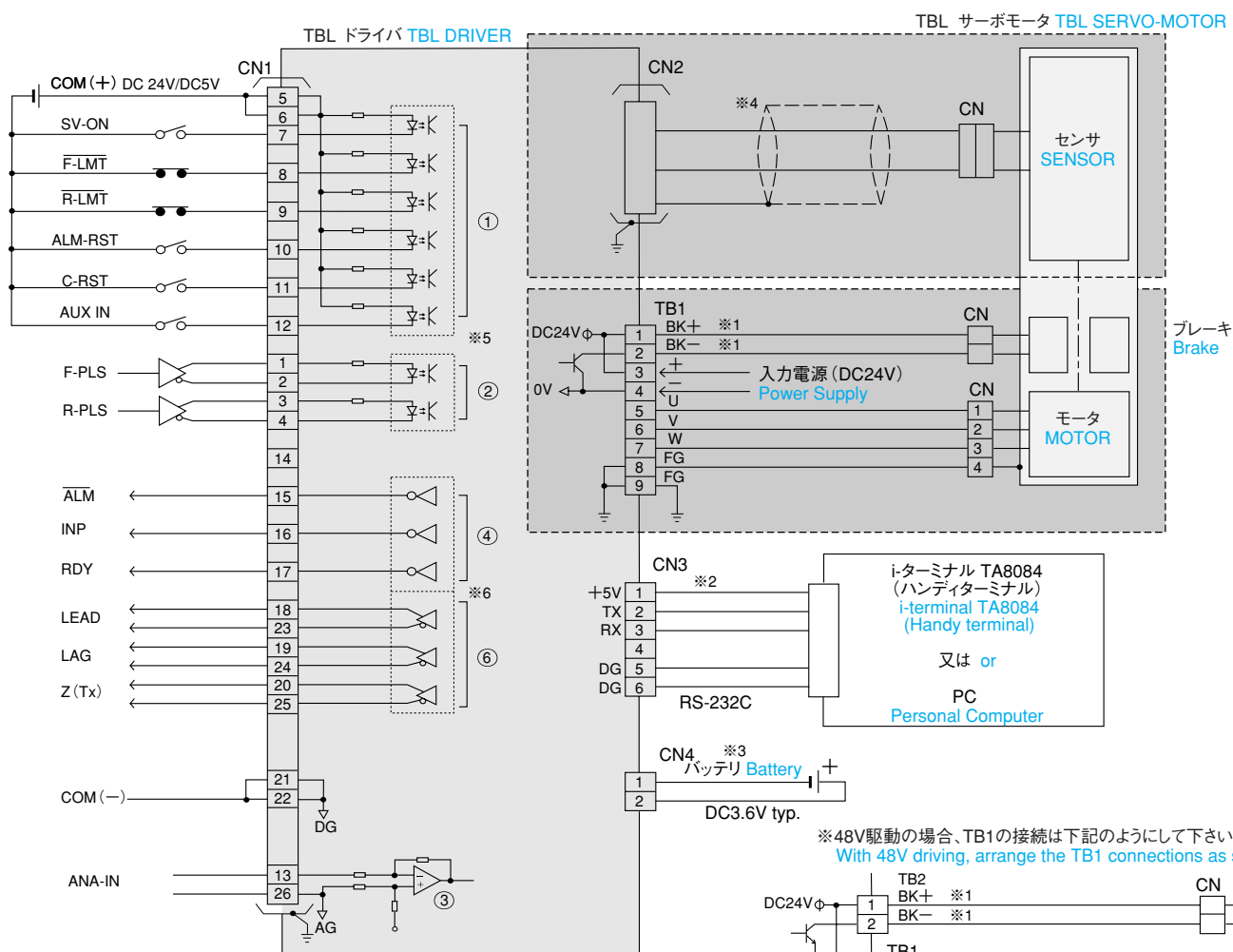
センサタイプ別接続 Sensor type-specific connections
